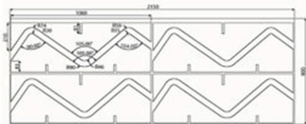
Figura 10 Libración molde lamina
