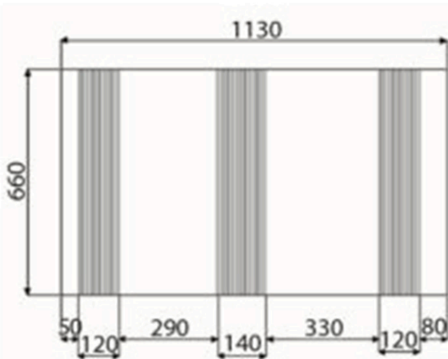
Figura 11 Ranurado del molde y contramolde
